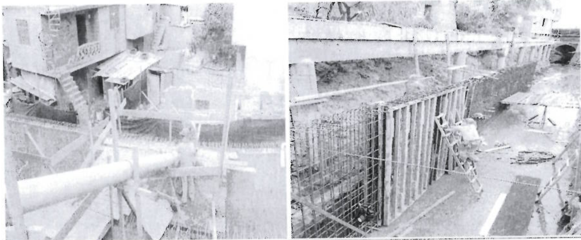
IMAGEN N° 09: Verificación de la parte Estructural, así como el cuidado necesario del doblado de los mismos y el trenzado de acuerdo a las especificaciones técnicas en la progresiva 0+450.
