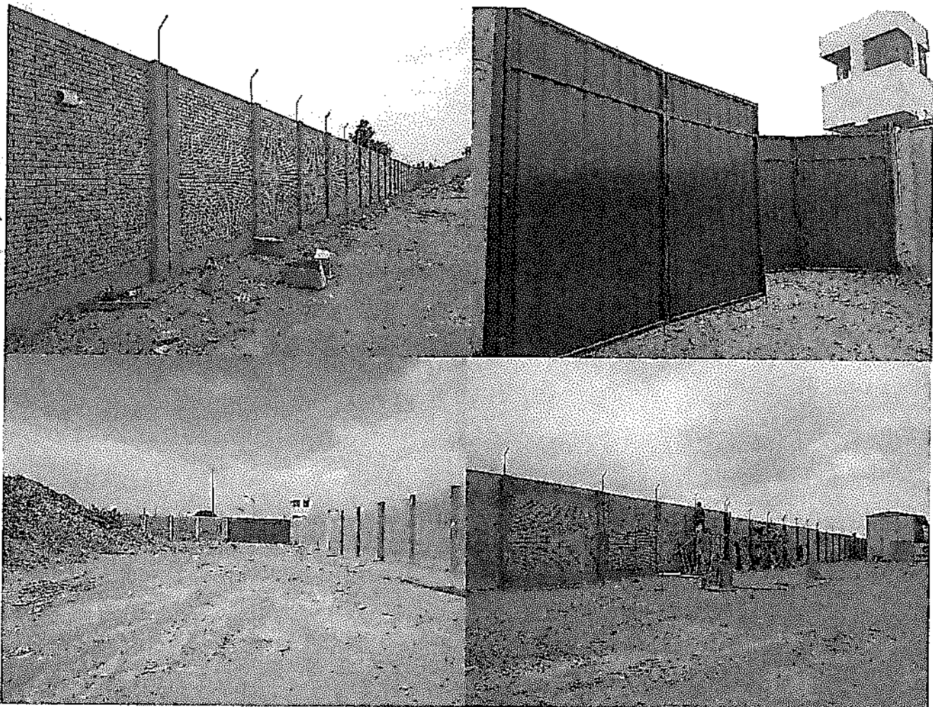
Fotografías de avance de Construcción del Cerco Perimétrico mes de noviembre Fuente: UEI COEN (noviembre 2019)
